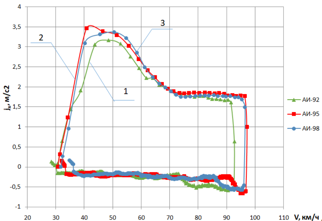
Рисунок 8. График зависимости ускорения от скорости при разгоне и выбеге автомобиля Toyota Chaser на бензине разных марок по ровному асфальтобетонному покрытию
