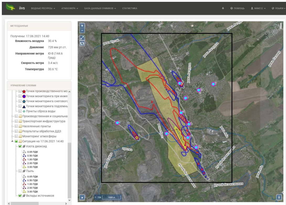
Рисунок 3. Интерфейс ПАК с отображением изолинии поля суммарных приземных концентраций
