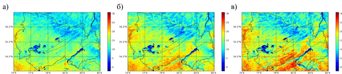
Рисунок 8. Распределение средней разности дневной и ночной температур в пикселе за периоды: а) 10.04–10.05.2010 г., б) 20.04–20.05.2010 г., в) 1.05–30.05.2010 г.
