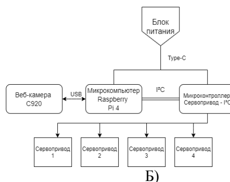
Рисунок 8: А) – Общий вид системы распознавания корнеклубнеплодов и луковец; Б) – Блок-схема системы управления комплексом машин послеуборочной обработки лука
