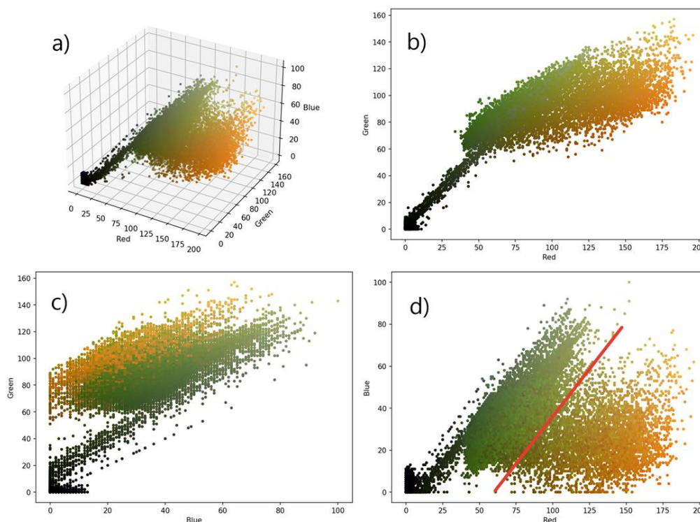
Рисунок 2. Диаграммы рассеяния RGB – а) трехмерная; б) двумерная, каналы G и R; в) двумерная, каналы G и B; г) двумерная, каналы B и R с ограничителем диапазонов
