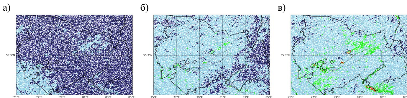
Рисунок 7. Распределение средней ночной температуры в пикселе за периоды:
