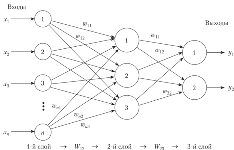
Рисунок 3. Многослойный перцептрон
