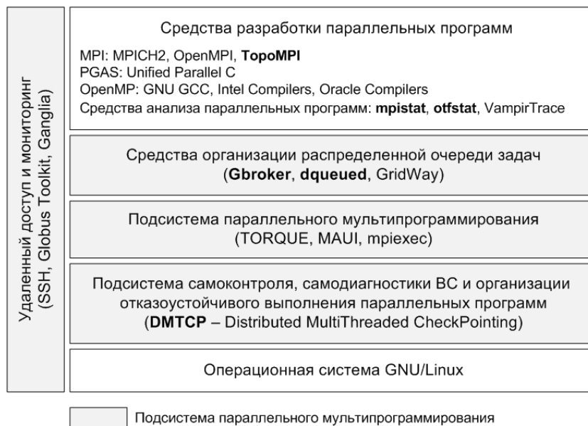
Рис. 2: Программное обеспечение пространственно-распределенной мультикластерной вычислительной системы
