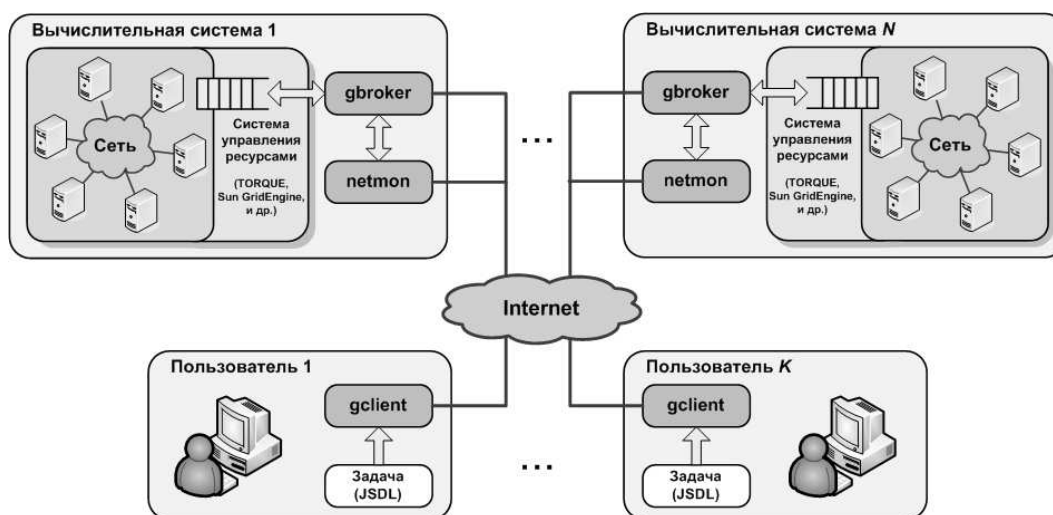
Рис. 3: Функциональная структура пакета GBroker
