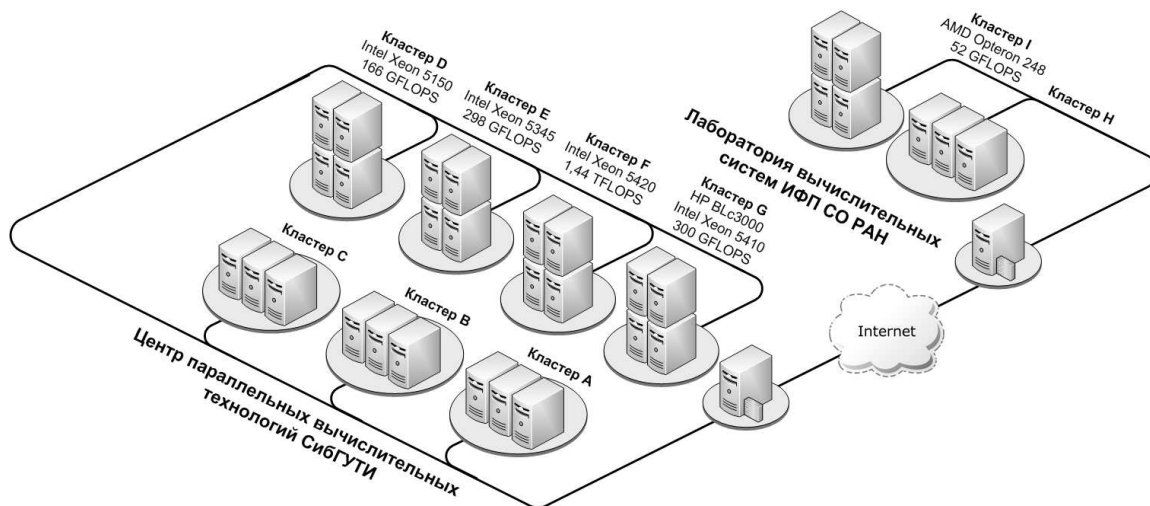
Рис. 1: Конфигурация пространственно-распределенной мультикластерной вычислительной системы
